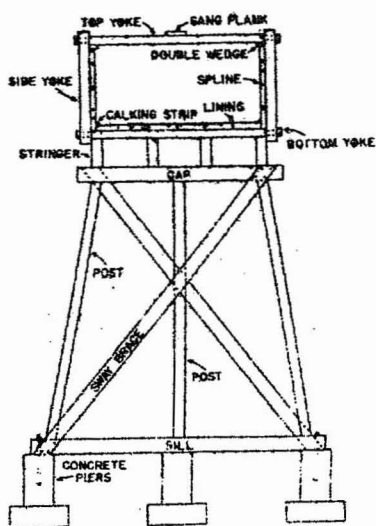
(D) FLUME CONSTRUCTION
